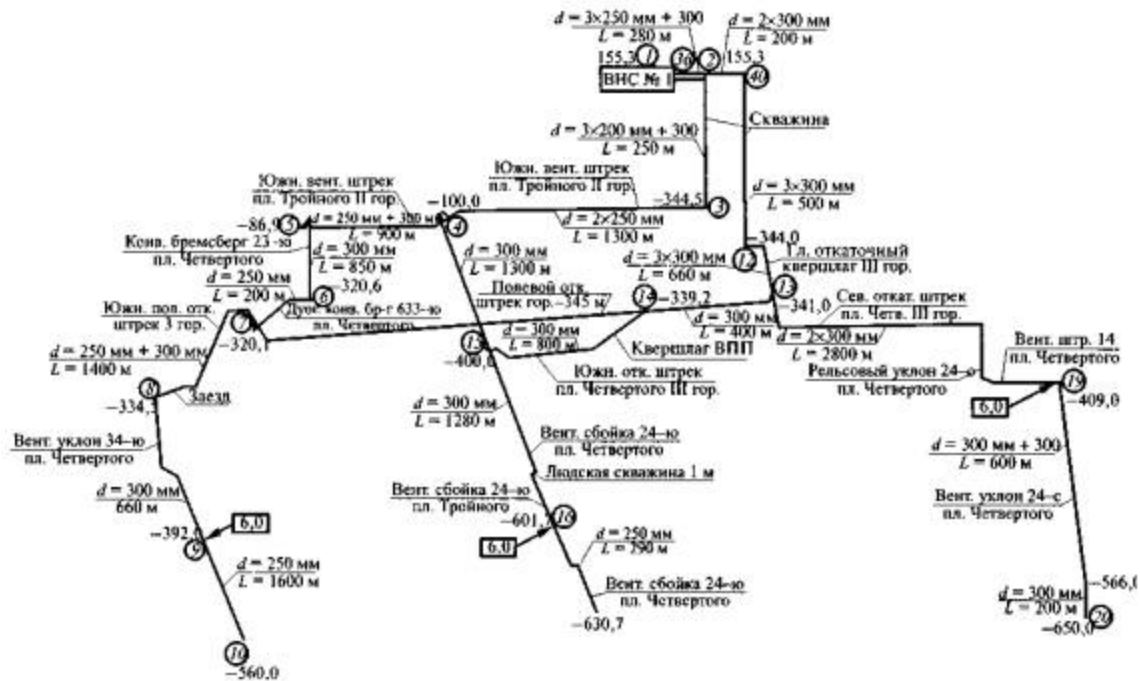
Рис. 8. Расчетная схема дегазационных трубопроводов шахты «Заполярная» (ОАО «Воркутауголь»):
