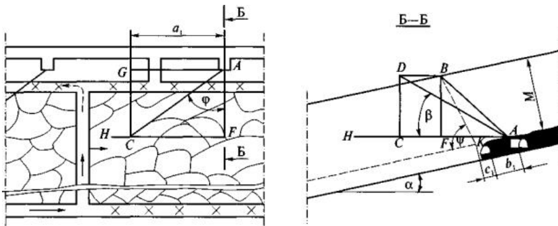
Рис. 1. Графическое определение параметров скважин, буримых на подрабатываемый пласт
