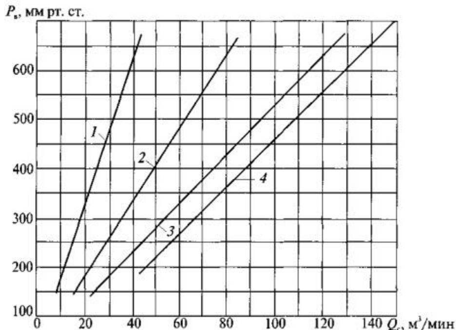
Рис. 3. Характеристика вакуум-насосов, работающих в режиме всасывания: 1 - отдельно работающий насос с номинальной производительностью 50 \text{ м}^3/\text{мин} ; 2 - два насоса с номинальной производительностью 50 \text{ м}^3/\text{мин} , работающие параллельно; 3 - три насоса с номинальной производительностью 50 \text{ м}^3/\text{мин} , работающие параллельно; 4 - отдельно работающий насос с номинальной производительностью 150 \text{ м}^3/\text{мин}
