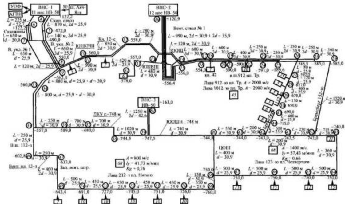
Рис. 7. Расчетная схема дегазационных трубопроводов шахты «Северная» (ОАО «Воркутауголь»):
