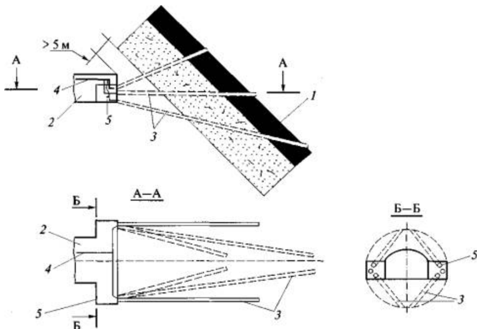
Рис. 2. Схема дегазации газоносного массива при вскрытии квершлагом: 1 - угольный пласт; 2 - квершлаг; 3 - скважина; 4 - дегазационный трубопровод; 5 - ниша
