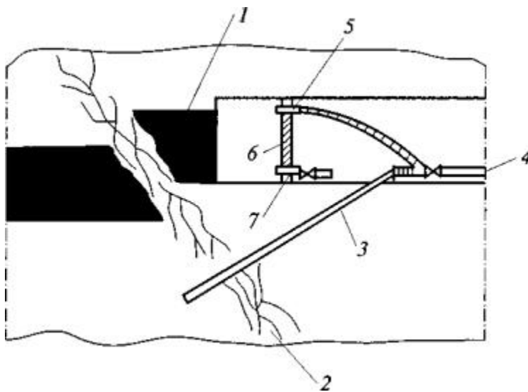
Рис. 2. Схема извлечения метана из суфлярных трещин средствами дегазации путем бурения скважин и возведения изолирующей забой перемычки: 1 - угольный пласт; 2 - геологическое нарушение; 3 - скважина; 4 - газопровод; 5 - труба для отвода газов; 6 - перемычка; 7 - труба с вентилем для слива воды
