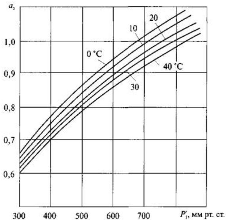
Рис. 4. Определение поправочного коэффициента a_3
