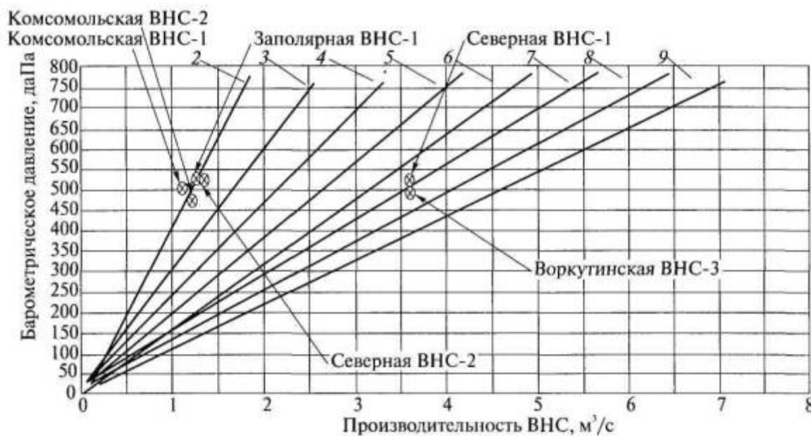
Рис. 6. Характеристики вакуум-насосных станций
