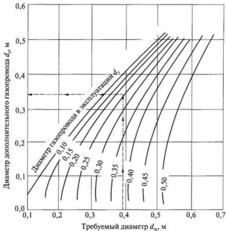
Рис. 5. Определение диаметра дополнительного газопровода
