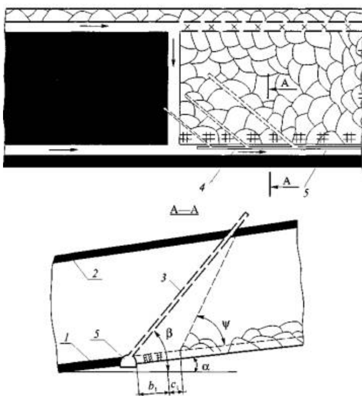
Рис. 2. Схема дегазации подрабатываемых пологих пластов скважинами, пробуренными из поддерживаемой за лавой выработки (схема 2): 1 - разрабатываемый пласт; 2 - подрабатываемый пласт; 3 - дегазационная скважина; 4 - газопровод; 5 - выработка, поддерживаемая за лавой; а - угол падения пласта; у - угол разгрузки пород кровли; б - угол возвышения скважины; b_1 - ширина целика (охранная зона); c_1 - резерв, учитывающий возможное отклонение скважины от заданного направления
