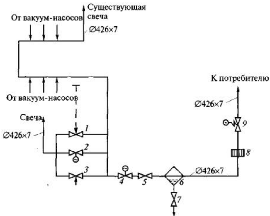
Рис. 1. Упрощенная технологическая схема газопроводов ВНС:
