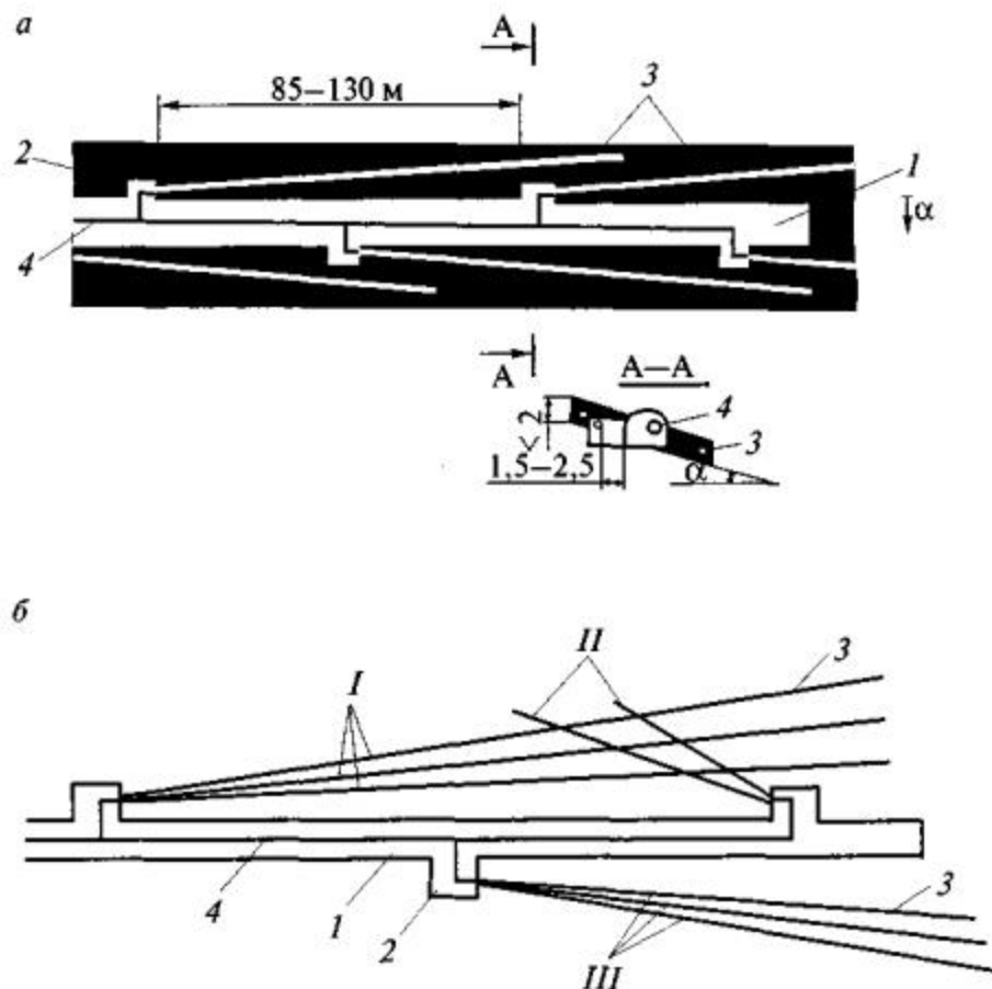
Рис. 5. Схема дегазации пласта барьерными скважинами: а - одиночные скважины; б - пересекающиеся скважины; I и II - серии пересекающихся барьерных скважин; III - серия барьерных скважин; 1 - штрек; 2 - камера; 3 - скважина; 4 - газопровод; а - угол падения пласта
