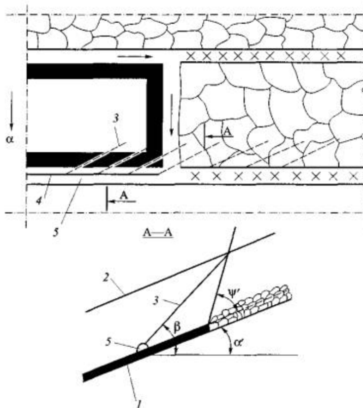
Рис. 3. Схема дегазации подрабатываемого пласта скважинами, пробуренными навстречу движущемуся очистному забою из погашаемой за лавой выработки (схема 3):
