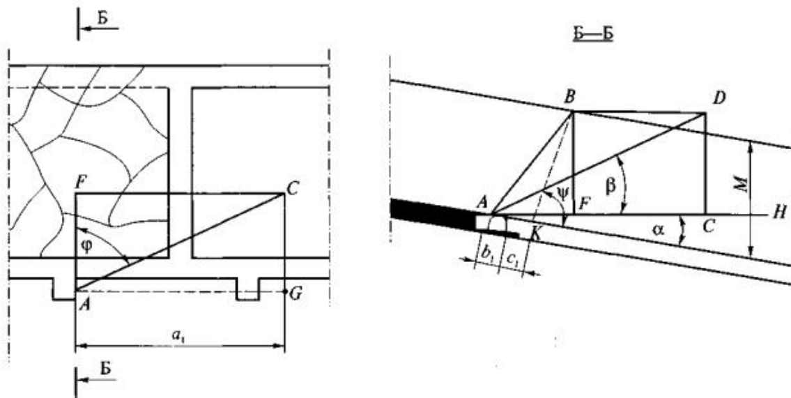
Рис. 3. Графическое определение параметров скважин, буримых из поддерживаемой за лавой выработки вслед очистному забою
