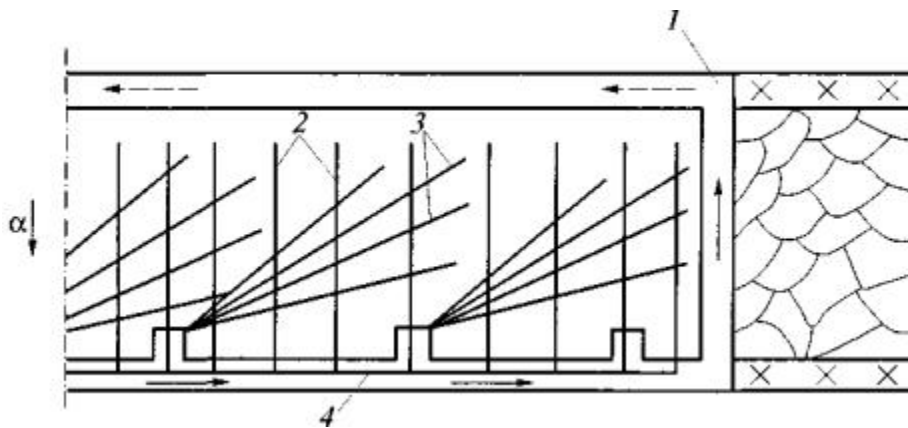
Рис. 11. Схема дегазации пласта параллельными и веерными, ориентированными на очистной забой скважинами:
