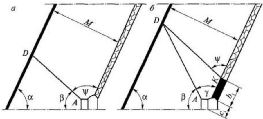
Рис. 1. Схема к определению направления скважины, буримой из откаточного штрека на вышележащий сближенный пласт в плоскости, нормальной к простираанию пласта:
