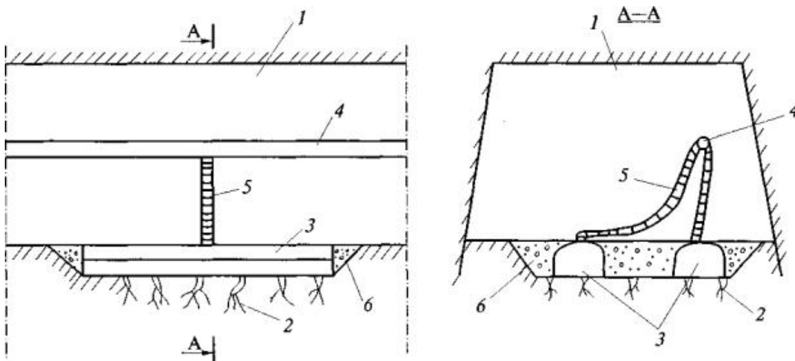
Рис. 1. Схема отвода суфлярных газов с помощью каптажных колпаков: 1 - выработка; 2 - массив угля или пород с суфлярными трещинами; 3 - каптажный колпак; 4 - дегазационный трубопровод; 5 - гибкий шланг; 6 - подушка, герметизирующая колпак
