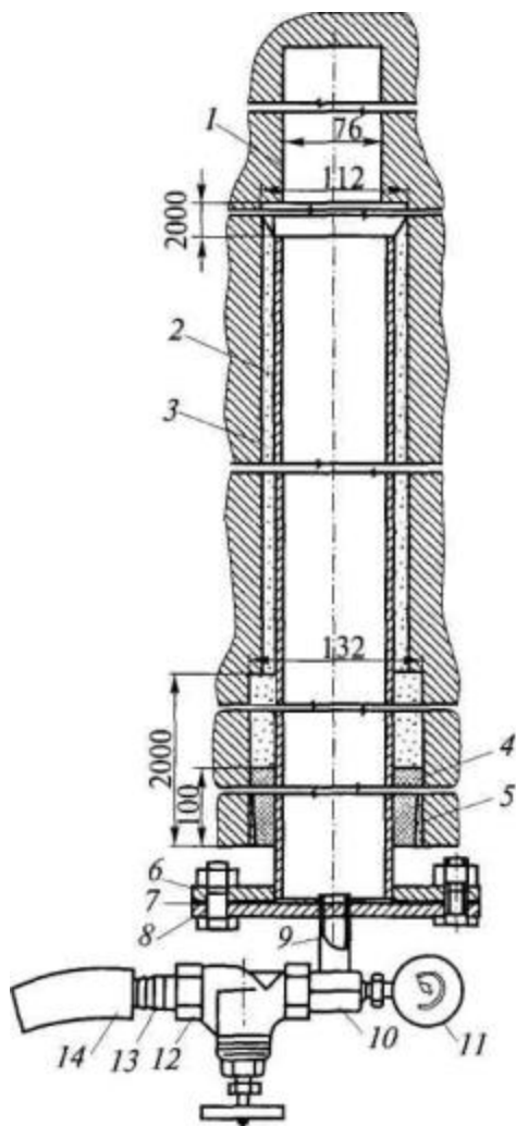
Рис. 2. Приспособление для контроля герметичности скважины:
