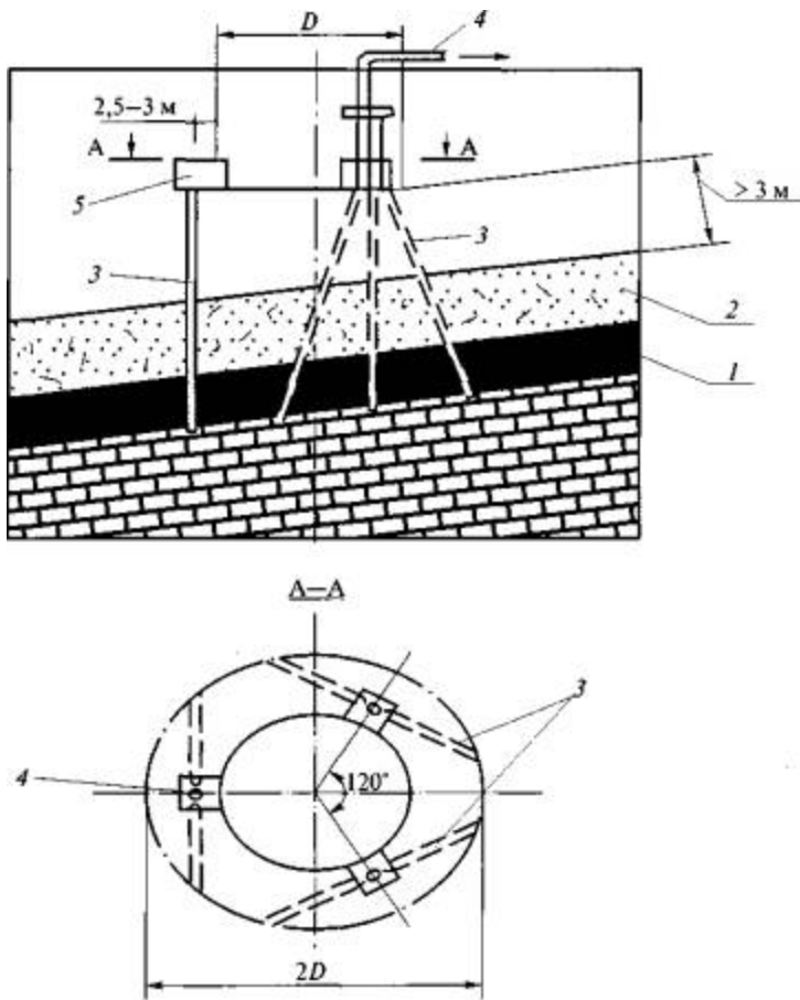
Рис. 1. Схема дегазации газоносного массива при проходке вертикальных выработок:
