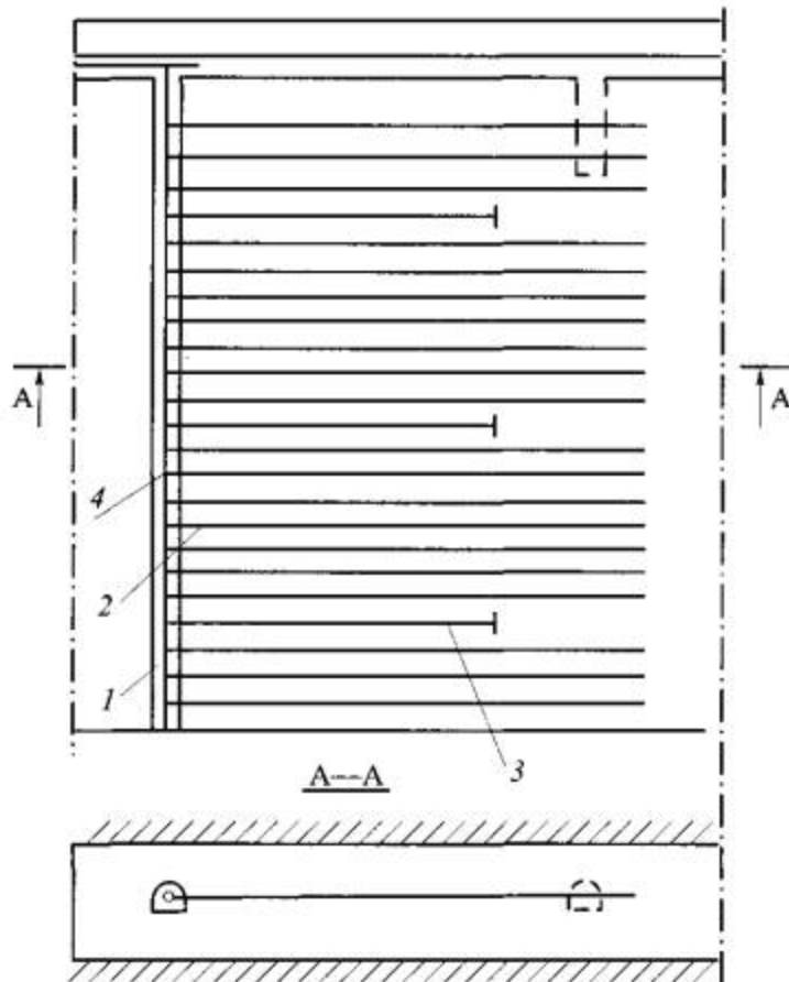
Рис. 17. Схема дегазации с предварительным гидроразрывом пласта через скважины, пробуренные из пластовой выработки:
