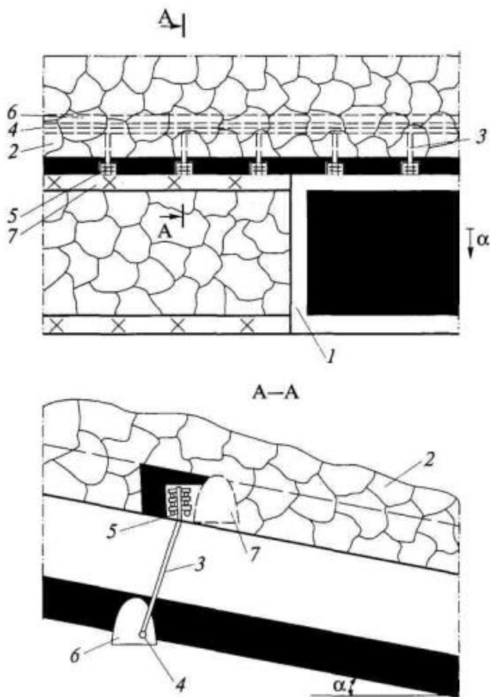
Рис. 3. Схема дегазации выработанного пространства перфорированными трубами с использованием сбоечных скважин:
