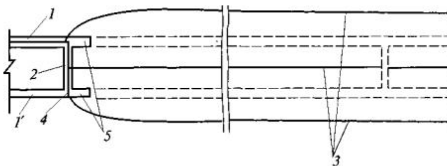
Рис. 6. Схема дегазации пласта длинными ограждающими скважинами направленного бурения: 1, 1' - выработки; 2 - сбойка; 3 - скважины направленного бурения; 4 - дегазационный трубопровод; 5 - забои спаренных выработок
