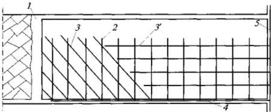
Рис. 9. Схема дегазации угольных пластов при ограниченных возможностях буровой техники:
