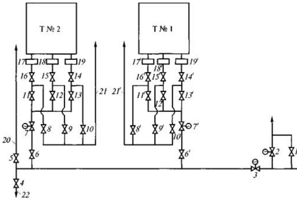
Рис. 2. Упрощенная технологическая схема газопроводов АГВН:
