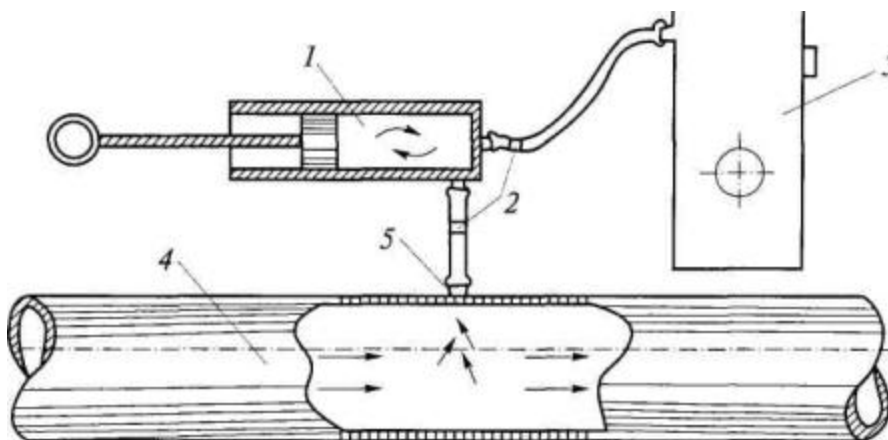
Рис. 2. Схема отбора проб газовой смеси:
