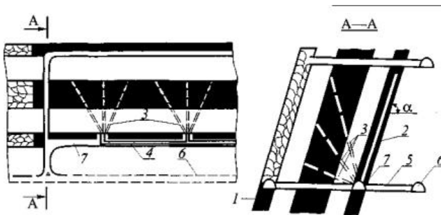
Рис. 15. Схема дегазации свиты крутых пластов скважинами, пробуренными веером вкрест одного пласта и в плоскости другого: 1 - обрабатываемый пласт; 2 - пластовые дегазационные скважины; 3 - дегазационные скважины, пробуренные вкрест пласта; 4 - газопровод; 5 - квершлаг; 6 - полевой штрек; 7- откаточный штрек
