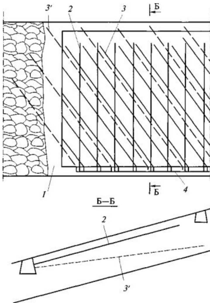
Рис. 13. Схема дегазации мощного пласта восстающими скважинами, пробуренными из выработок верхнего слоя (схема II):
