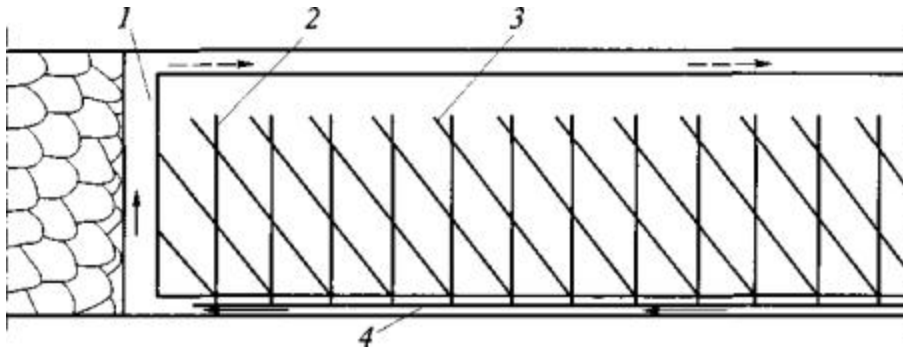
Рис. 10. Схема дегазации угольных пластов перекрещивающимися скважинами, пробуренными из конвейерной выработки:
