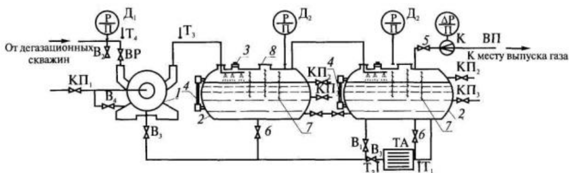
Рис. 4. Упрощенная технологическая схема передвижной дегазационной установки ПДУ-50:
