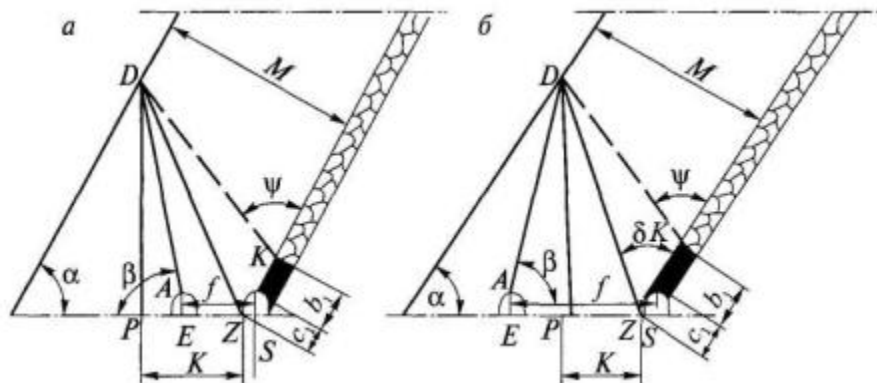
Рис. 3. Схема к определению параметров скважины, буримой из группового откаточного штрека на вышележащий сближенный пласт, в плоскости, нормальной к простиранию пласта и при наличии целика угля (бутовой полосы) над штреком: a - K > f ; b - K < f ; ( K = PZ ; f = ES )
