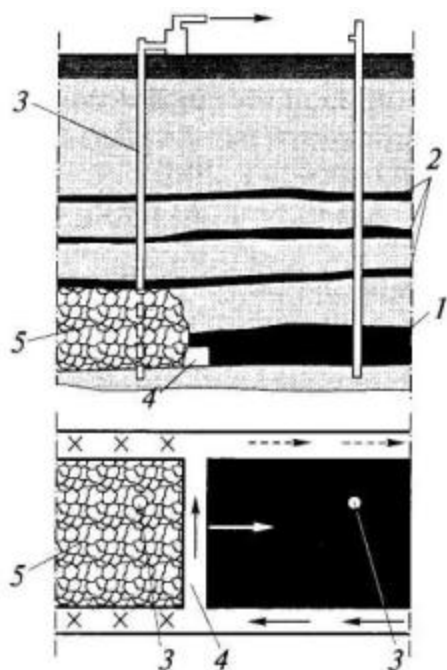
Рис. 1. Схема дегазации сближенных пластов и выработанного пространства скважинами, пробуренными с поверхности: 1 - разрабатываемый пласт; 2 - сближенные пласты; 3 - скважина; 4 - очистной забой; 5 - выработанное пространство
