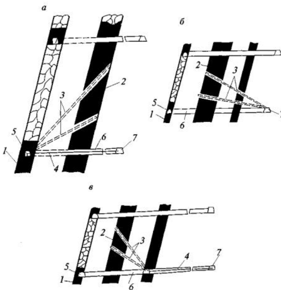
Рис. 1. Схема дегазации надрабатываемого крутого пласта скважинами, пробуренными веером вкрест его залегания:
