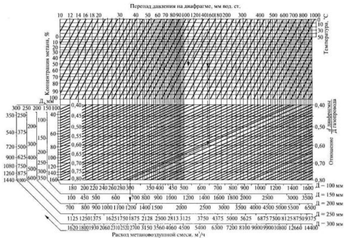
Рис. 6. Определение расхода газа Q_g, \text{м}^3/\text{ч}
