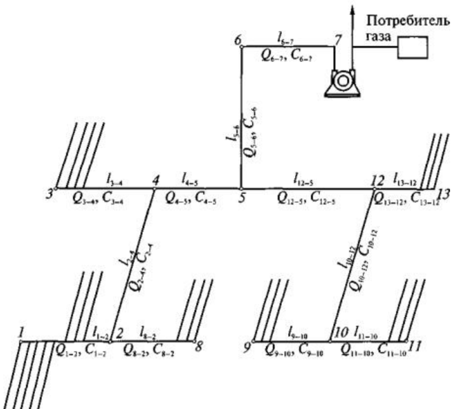
Рис. 1. Схема для расчета газопроводов
