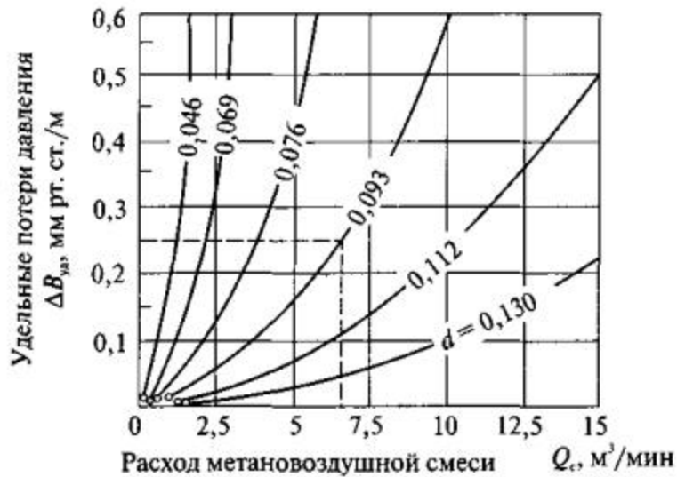
Рис. 2. Определение удельных потерь давления в скважине
