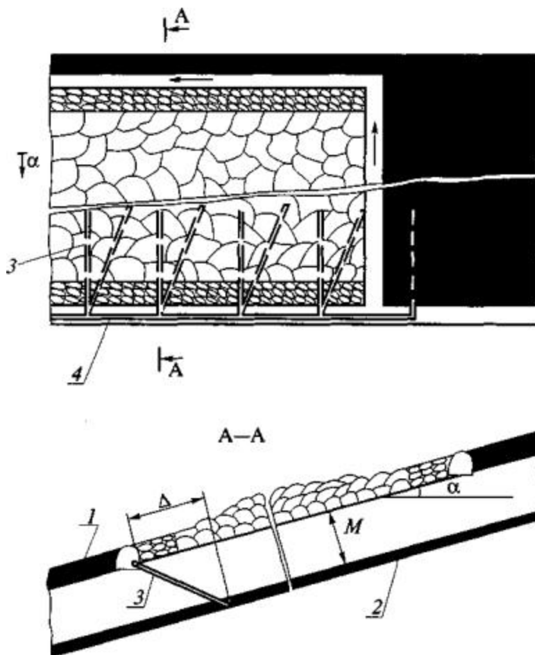
Рис. 2. Схема дегазации надрабатываемого пласта скважинами, пробуренными из поддерживаемой за лавой откаточной выработки:
