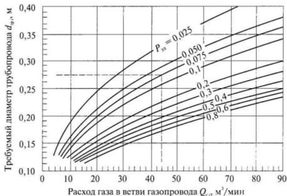
Рис. 4. Определение диаметра газопровода
