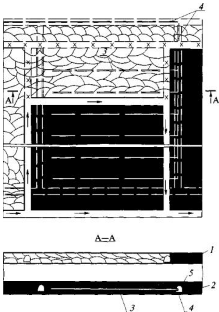
Рис. 3. Схема дегазации надрабатываемого угольного пласта пластовыми скважинами:
