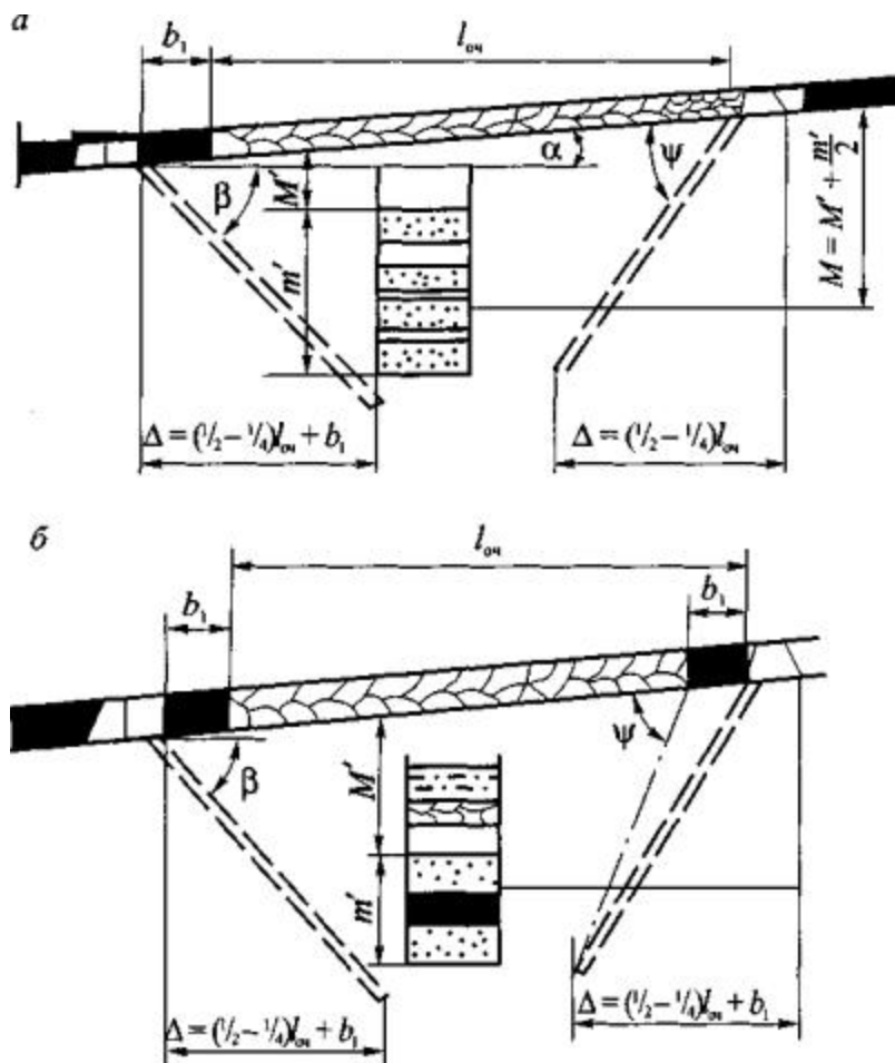
Рис. 1. Схемы дегазации надрабатываемой толщи горных пород: а - при отсутствии сближенного угольного пласта; б - при наличии сближенного угольного пласта; M' - расстояние по нормали между разрабатываемым пластом и дегазируемой толщей газосодержащих пород; m' - мощность дегазируемой толщи пород; \alpha - угол падения пласта; \psi - угол наклона скважины к горизонту; b_1 - протяженность зоны (ширина целика угля), препятствующей разгрузке горных пород; l_{оч} - длина лавы; \gamma_1 - угол разгрузки пород почвы
