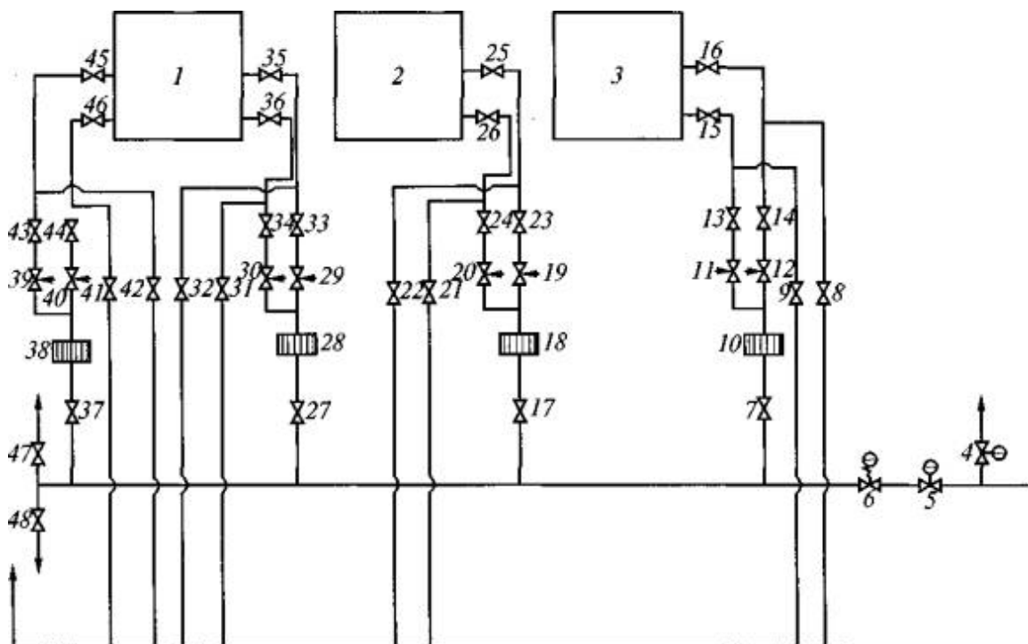
Рис. 3. Упрощенная технологическая схема газопроводов котельной (шахта «Комсомольская»):
